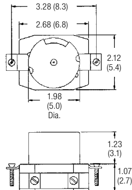
50A Receptacle
